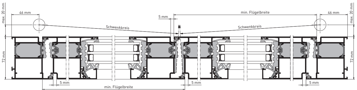
heroal D 72, représentation en coupe, capacité au déclenchement, cote d'espacement 5 mm
