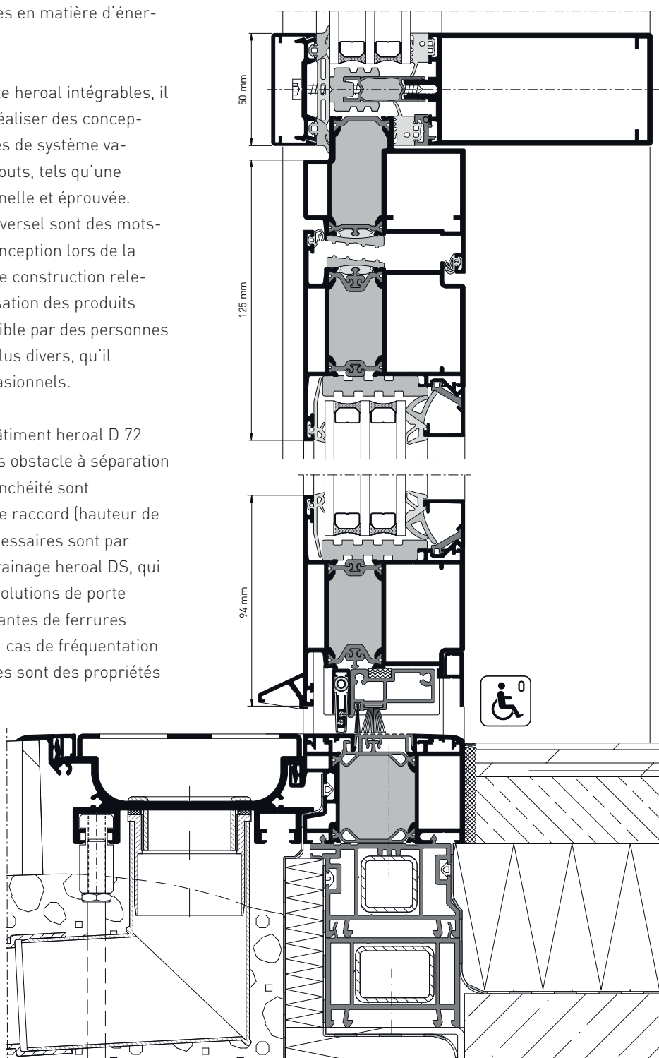
heroal D 72, représentation en coupe, intégration à la façade
