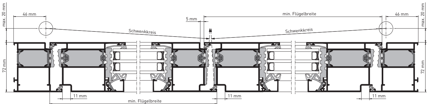
heroal D 72, représentation en coupe, capacité au déclenchement, cote d'espacement 11 mm
