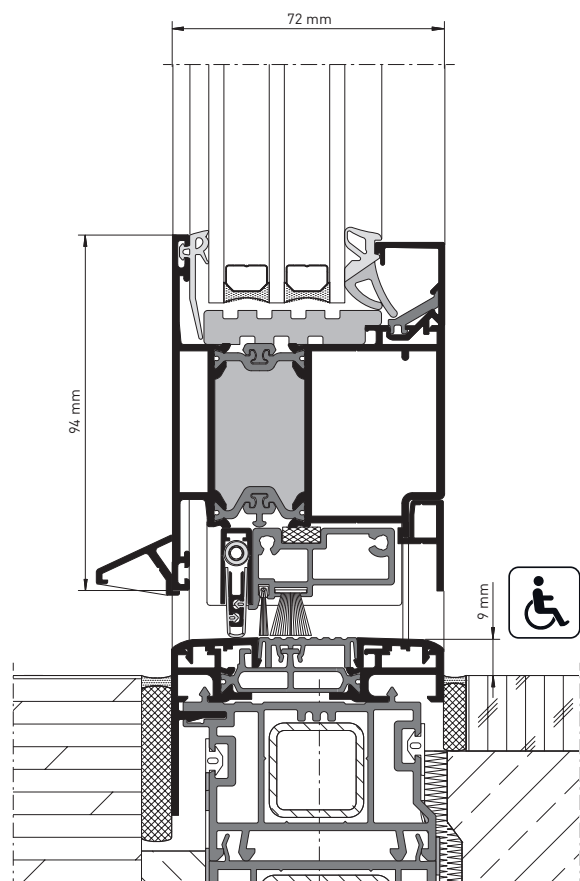
heroal D 72, représentation en coupe, avec accessibilité aux handicapés selon DIN 18040
